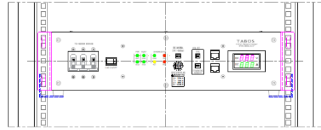
(참고) 19인치 표준랙 장착도 필요 력깊이 D=600mm, L형 선반 필요
