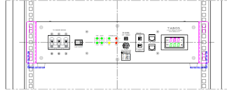
(참고) 19인치 표준랙 장착도 필요 랙깊이 D=600mm, L형 선반 필요
