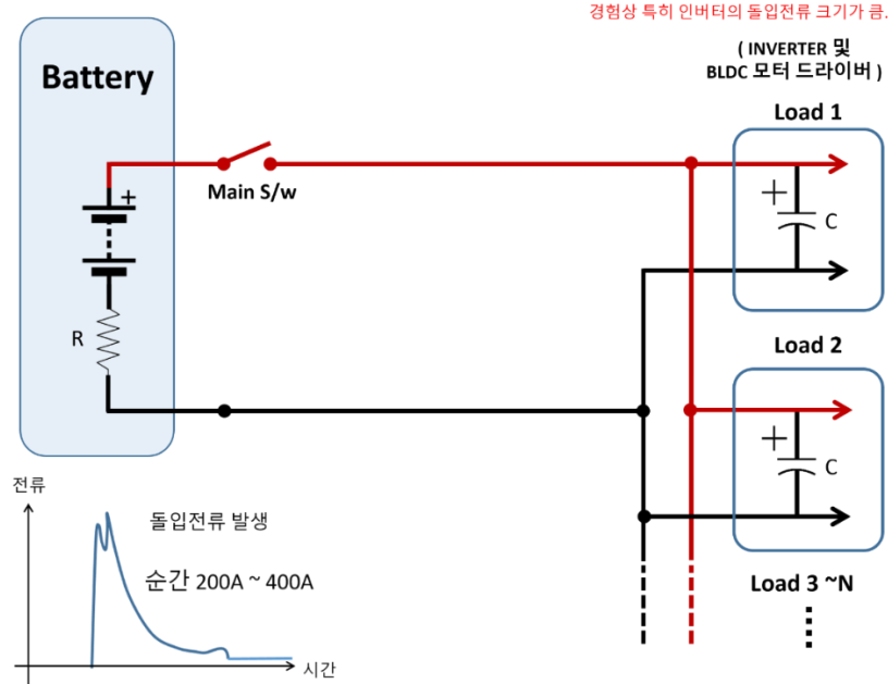
[그림 1] (아래) 일반적인 계통도
