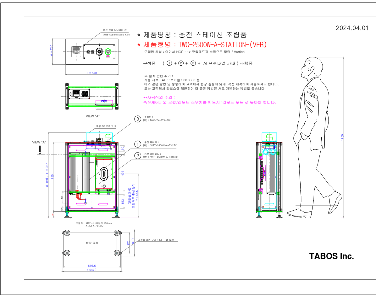
⑥-2 충전스테이션-A / 코일패드 수직
