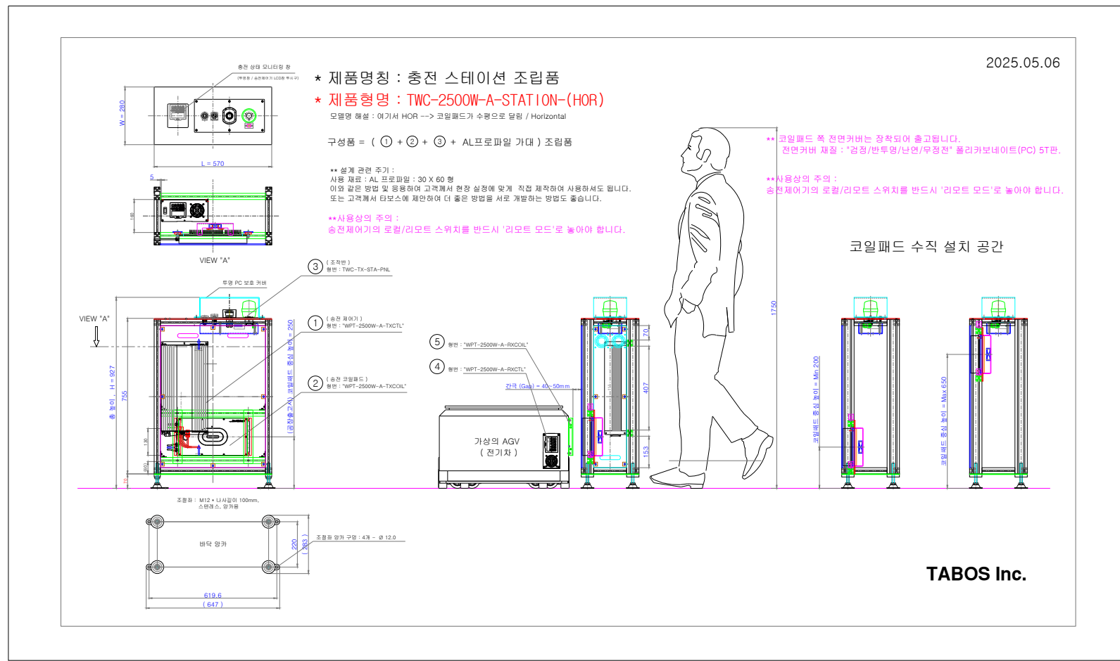
⑥-1 충전스테이션-A / 코일패드 수평
