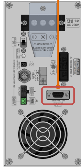
송전제어기(TX)
