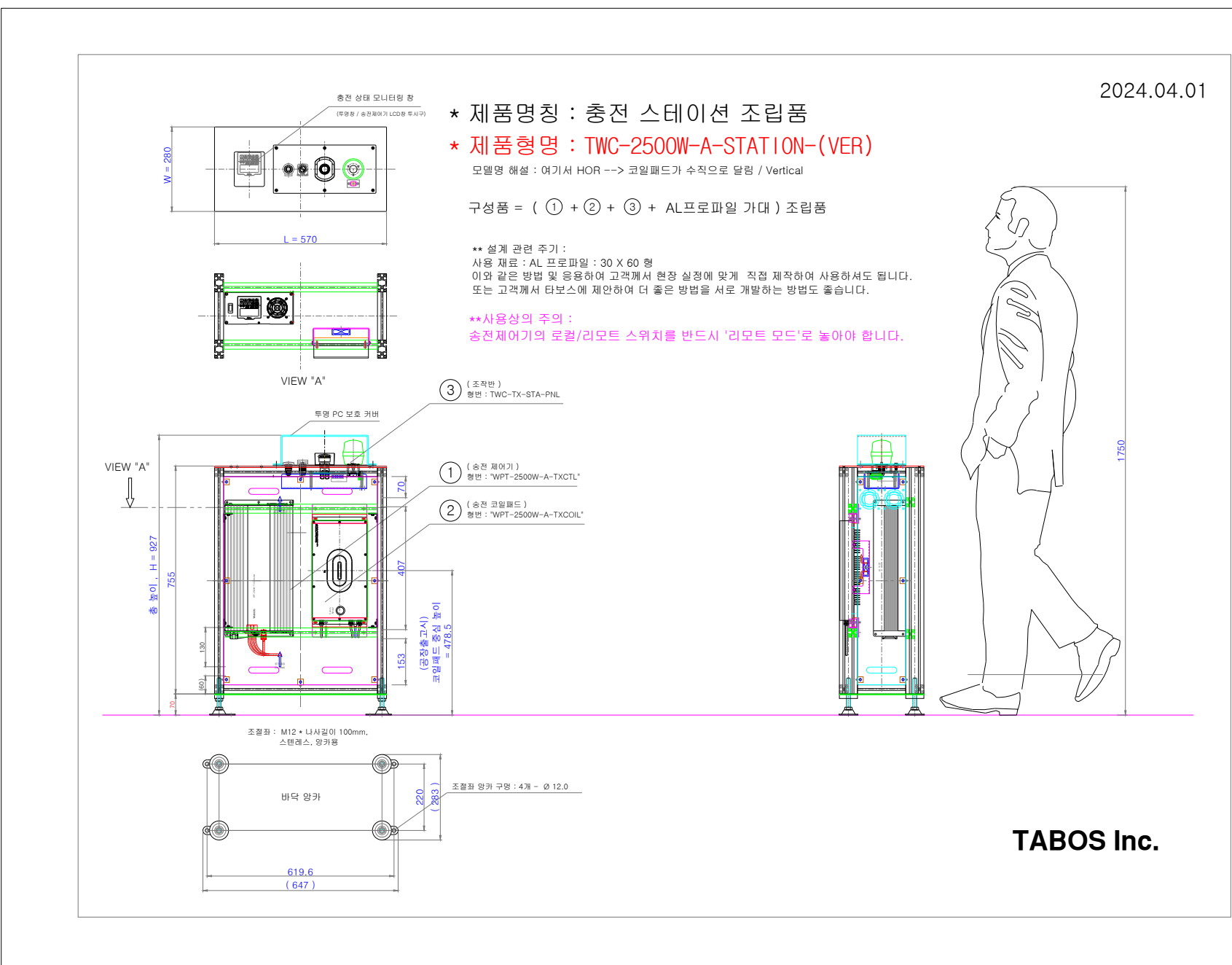
⑥-2 충전스테이션-A / 코일패드 수직
