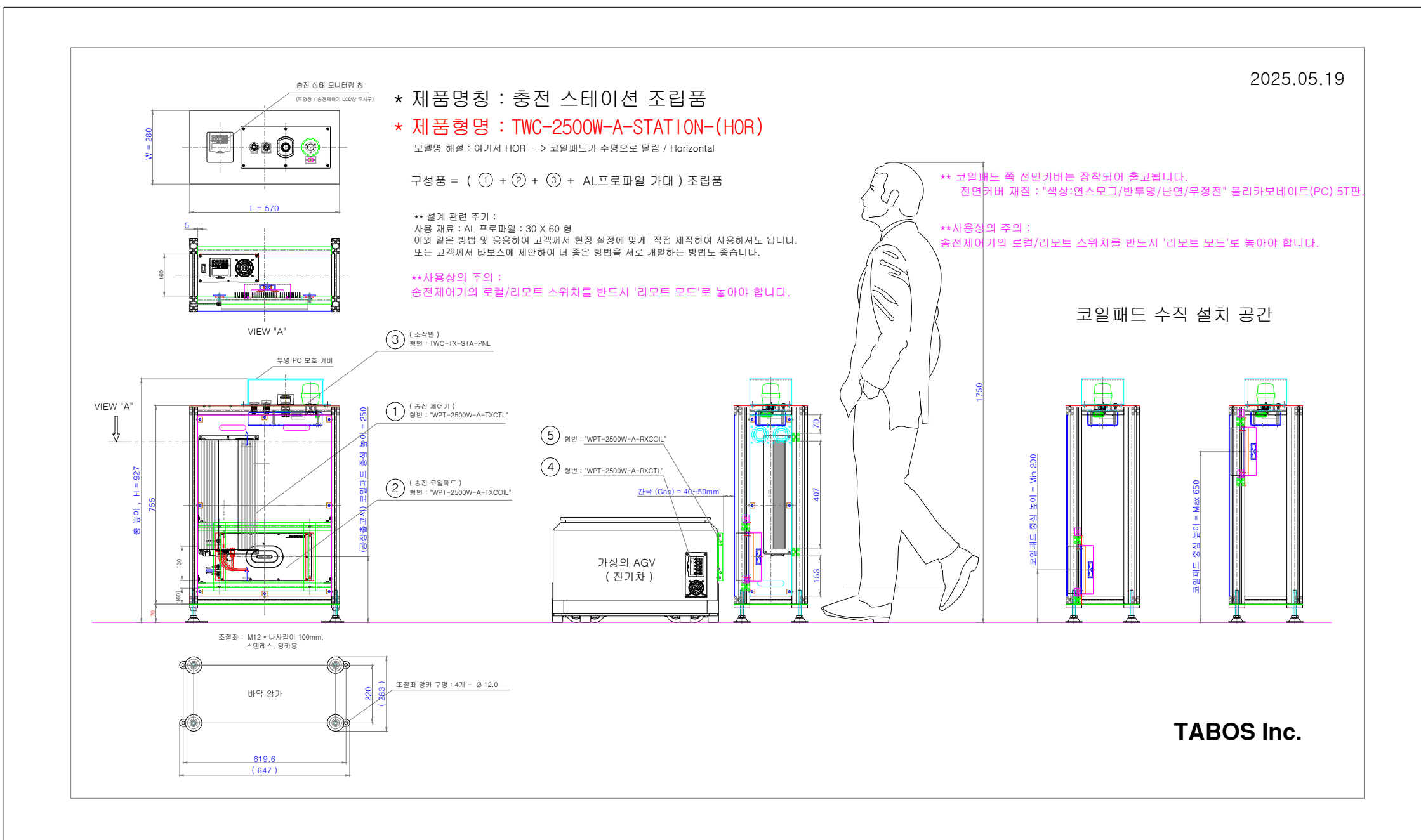
⑥-1 충전스테이션-A / 코일패드 수평
