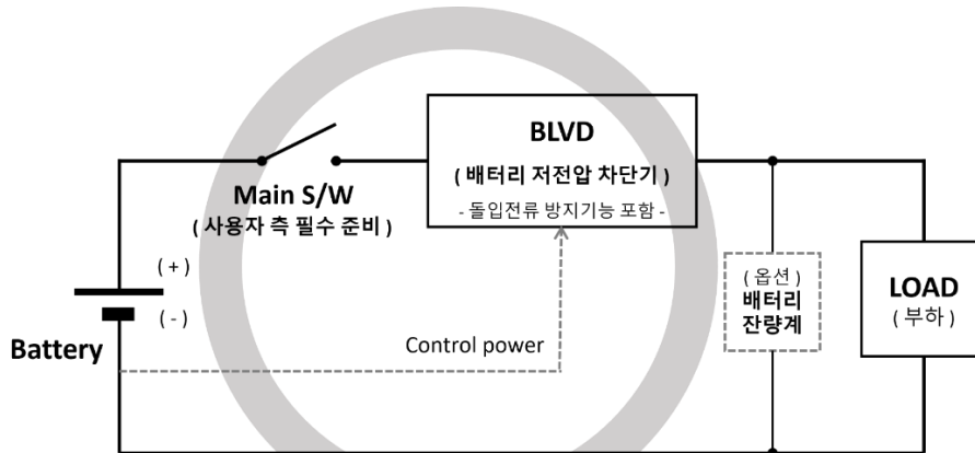
( 올바른 방법 )
