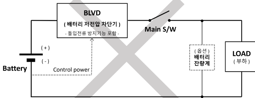
( 잘못된 방법 )
